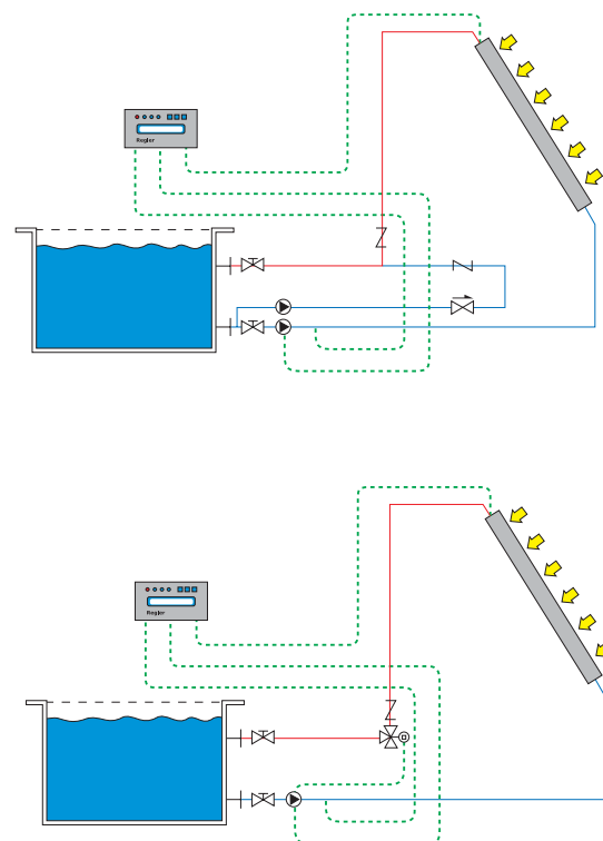
■ příklady instalace
